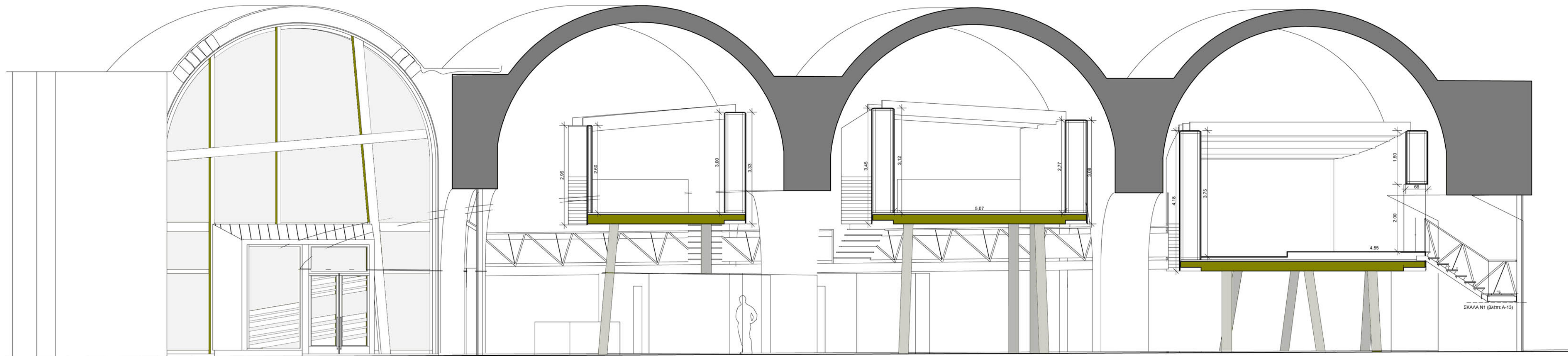
TOMH B-B'
